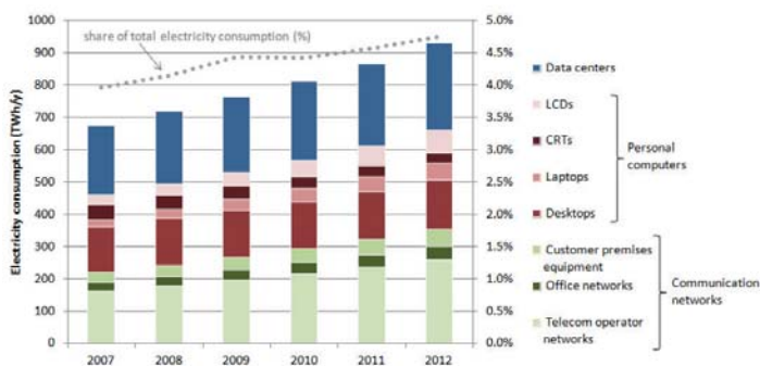
Figure 3: (Figure 3.1 du rapport [3]) Utilisation mondiale de l'électricité pour les différents secteurs des TIC, ainsi que la part totale dans la consommation sur la période 2007-2012 (4,7% en 2012).
