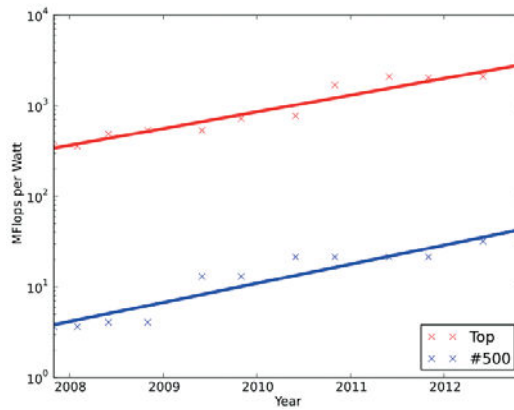
Figure 5: «Loi de Moore» projetée en Mflops/Watt (Wikipedia). [1 Mflops = 1 million d'opérations par seconde].
