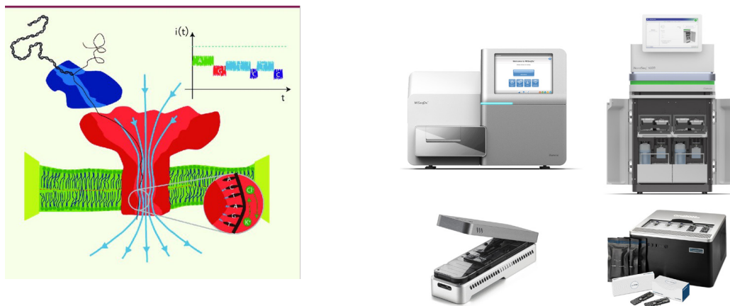
Figure 1.8 Séquençage
